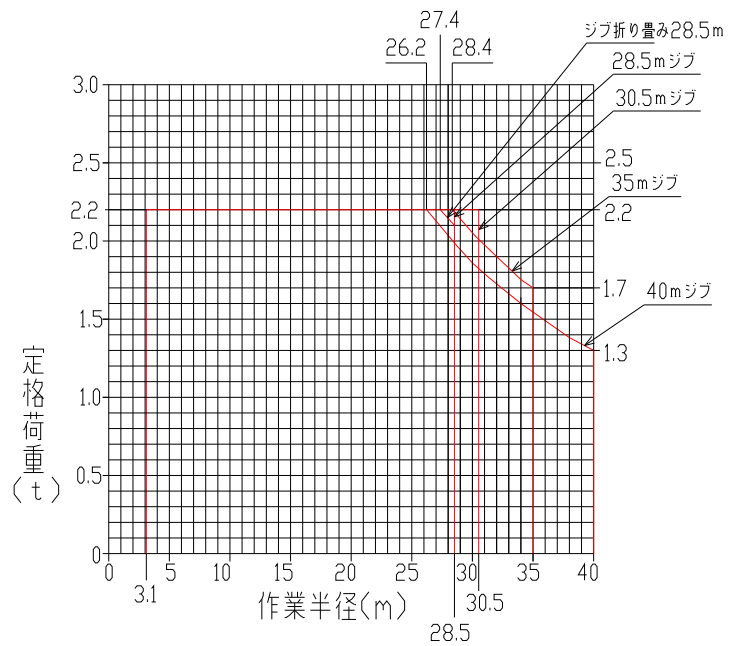
POTAIN IGOT70 定格荷重曲線 2本掛け
