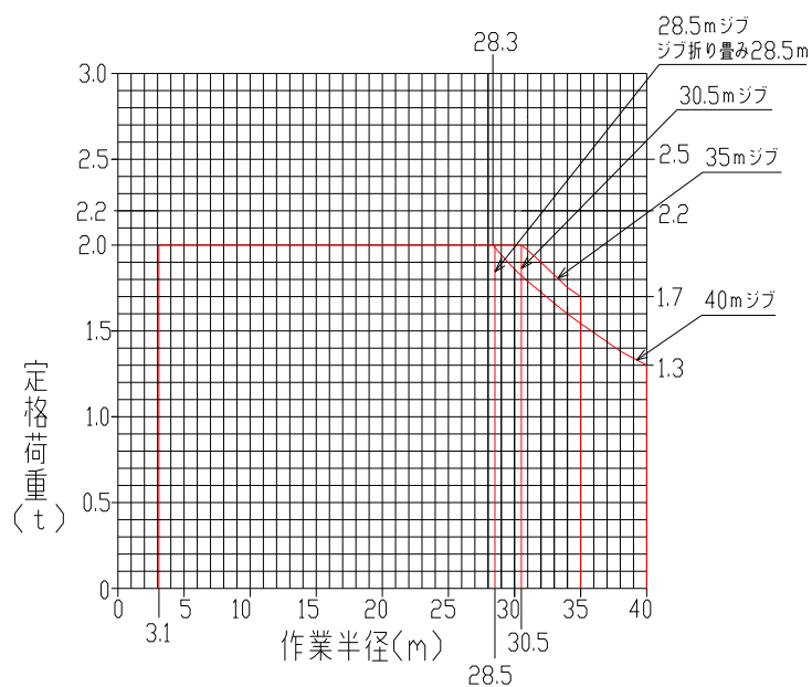
POTAIN IGOT70 定格荷重曲線 2本掛け
