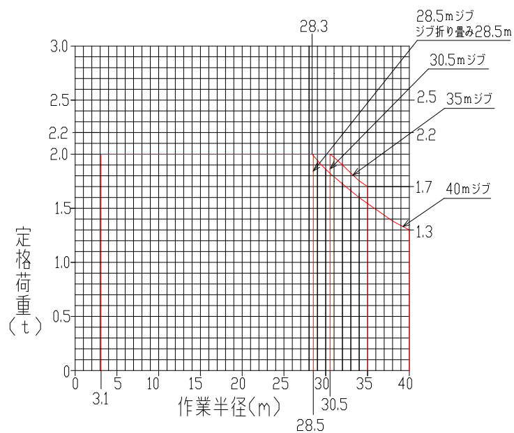
POTAIN IGOT70 定格荷重曲線 2本掛け
