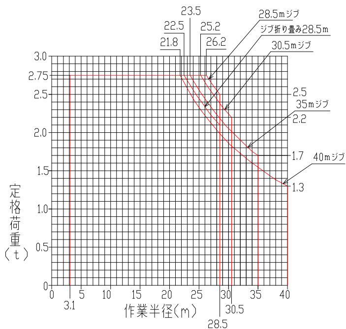
POTAIN IGOT70 定格荷重曲線 4本掛け
